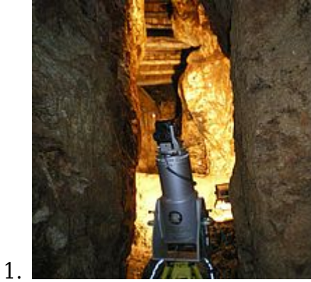
Terrestrischer Lasses scanner © Landesamt für Archäologie Sachsen
